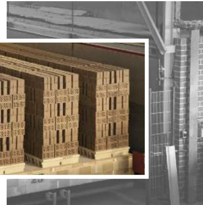
Einfahrt in den Vorwärmer
