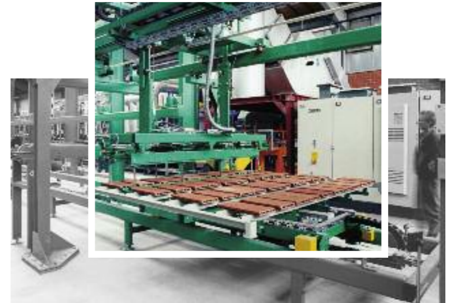
Transfer device Dispositivo de traslación
